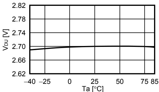
(5) V_{DU} - T_a
