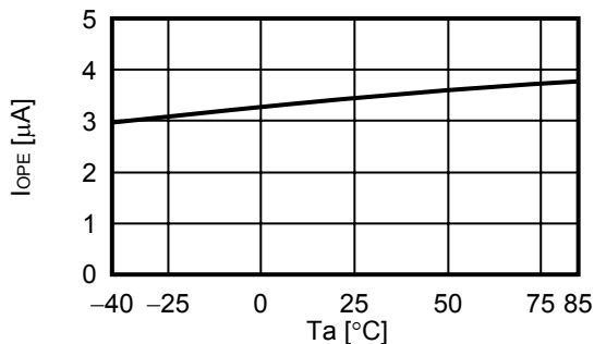
(1) I_{OPE} - T_a
