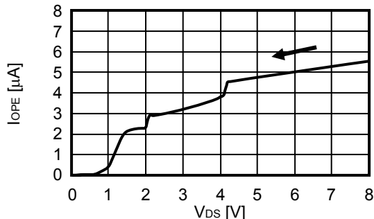
(2) I_{OPE} - V_{DS}
